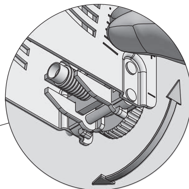
UWAGA! regulować przy mniejszym kącie otwarcia NOTE! adjust with a smaller opening angle ВНИМАНИЕ! Регулирование при малом угле открывания
