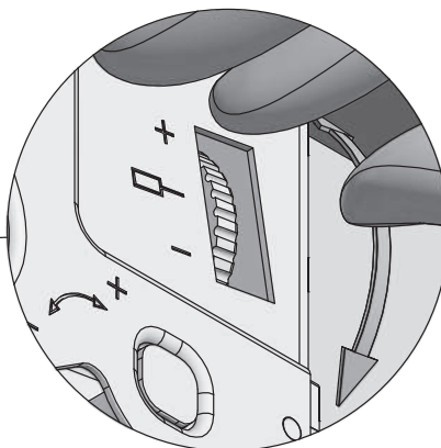
regulacja czasu domknięcia closing time adjustment регулировка времени закрывания
