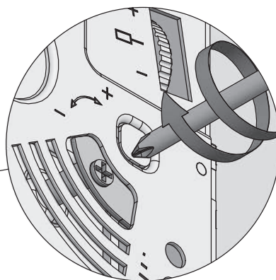
regulacja siły otwarcia opening force adjustment регулировка усилия при открывании
