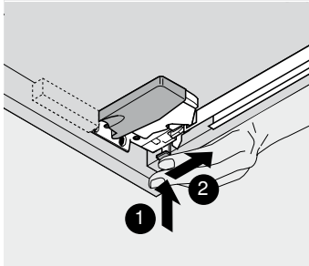
560H/566H/550H Ajuste altura + 3 mm
