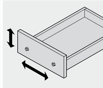
Ajuste de la altura y el lateral del herraje de ajuste del frente ± 2 mm
